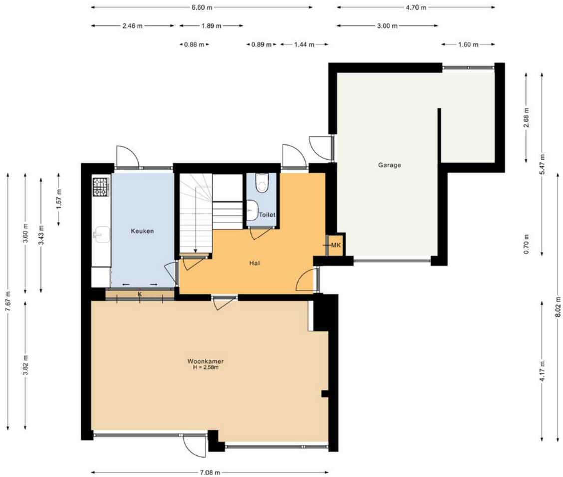
Begane grond Oranjelaan 83 Lisse
