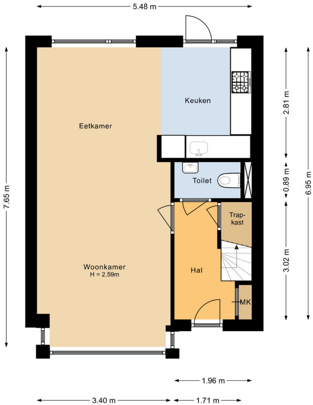
Begane grond
